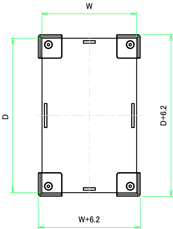
上カバー / Top cover
